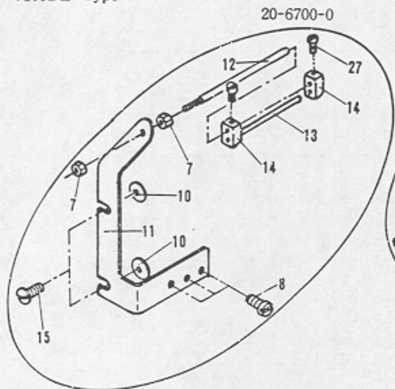
Tape guide
